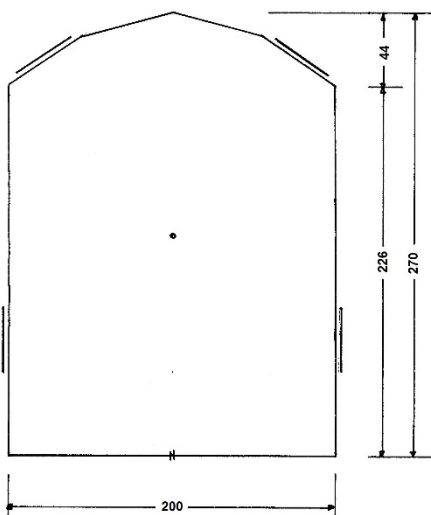
Grundriß Pyramidenzelt TROPIC MINI Art. 71 270 200
